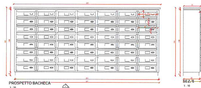
PROSPETTO BACHECA 1 : 10
