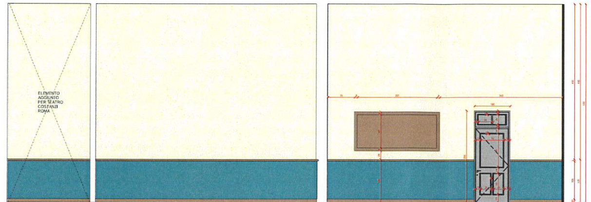
PROSPETTO UFFICIO PARETE DI FONDO 1 : 20
