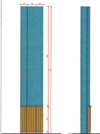
PROSP. ELEM. APRIBILE 1 : 20
