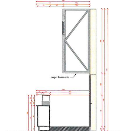
Section 000 1:20
