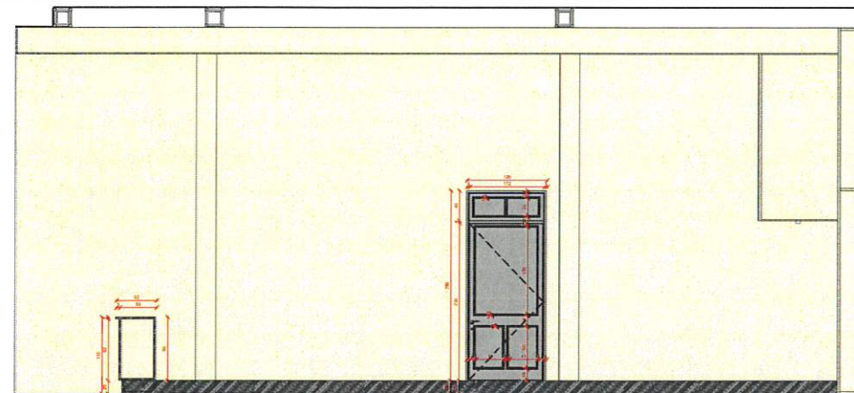
SEZIONE 4 1:20
