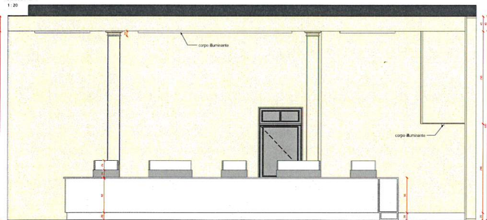
PROSPETTO BANCA ELEMENTO 1 1:20
